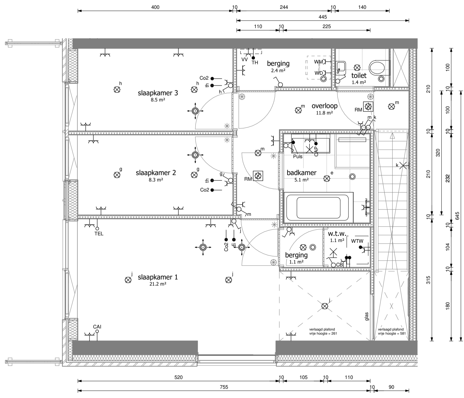
Eerste verdieping type A1a schaal 1 : 50
