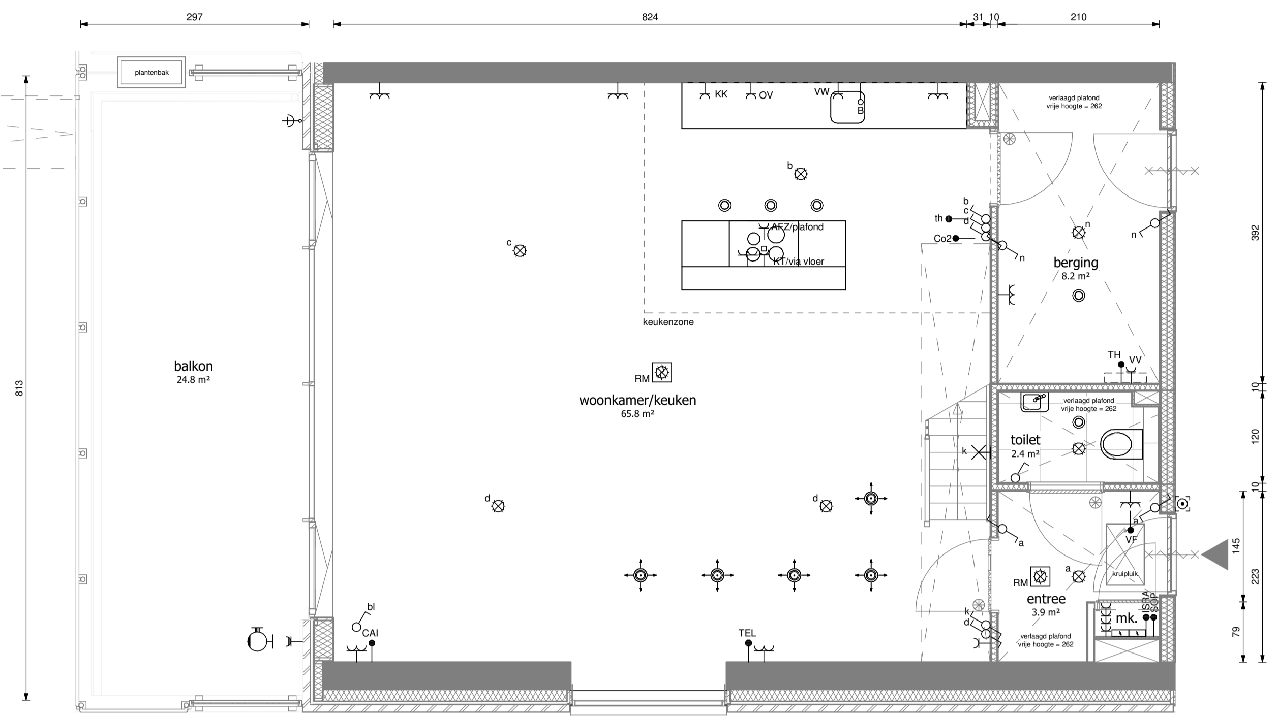
Begane grond type A1a schaal 1 : 50
