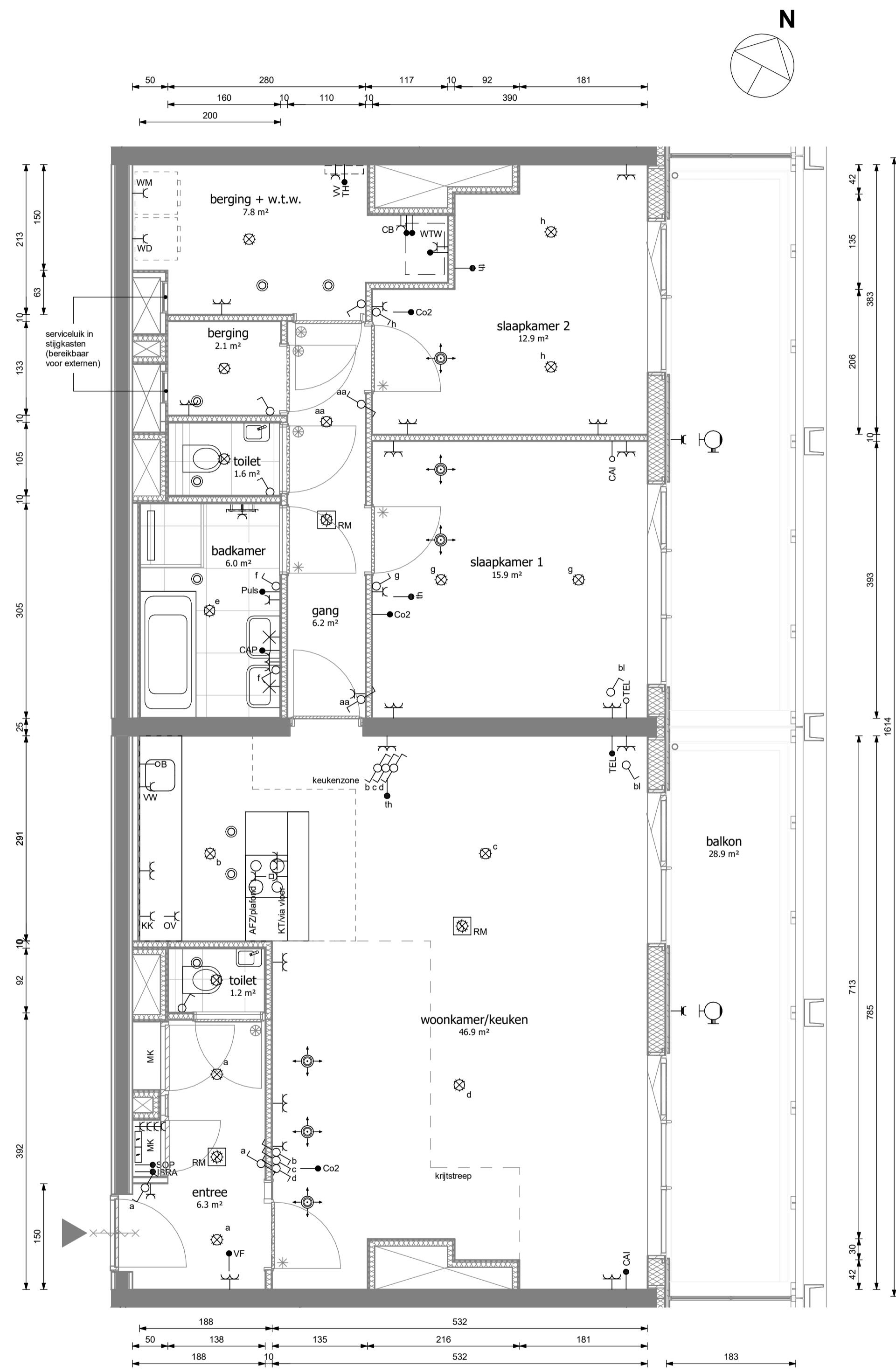
Type E10a schaal 1:50
