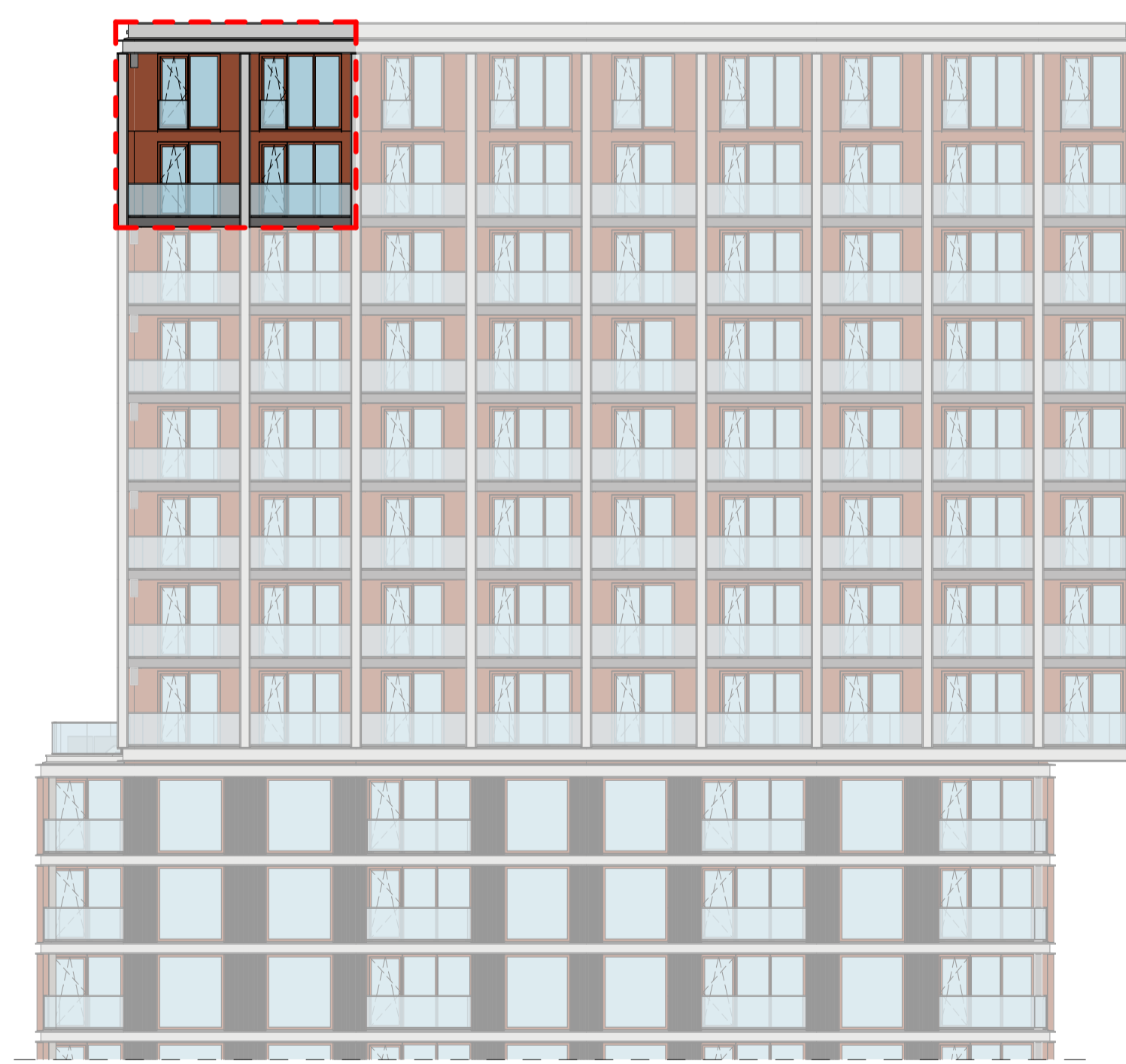
westgevel
