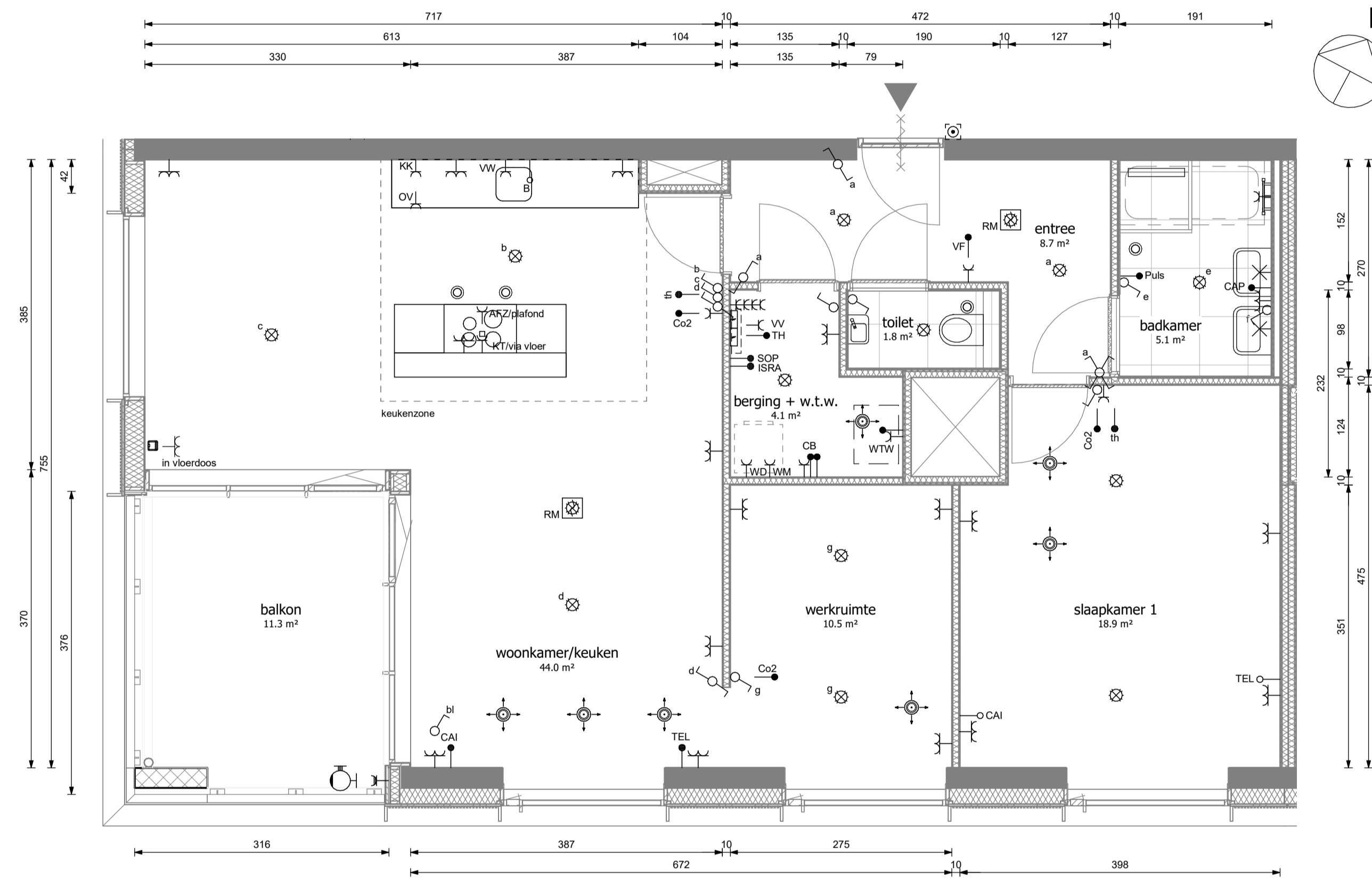
Type D1d schaal 1:50
