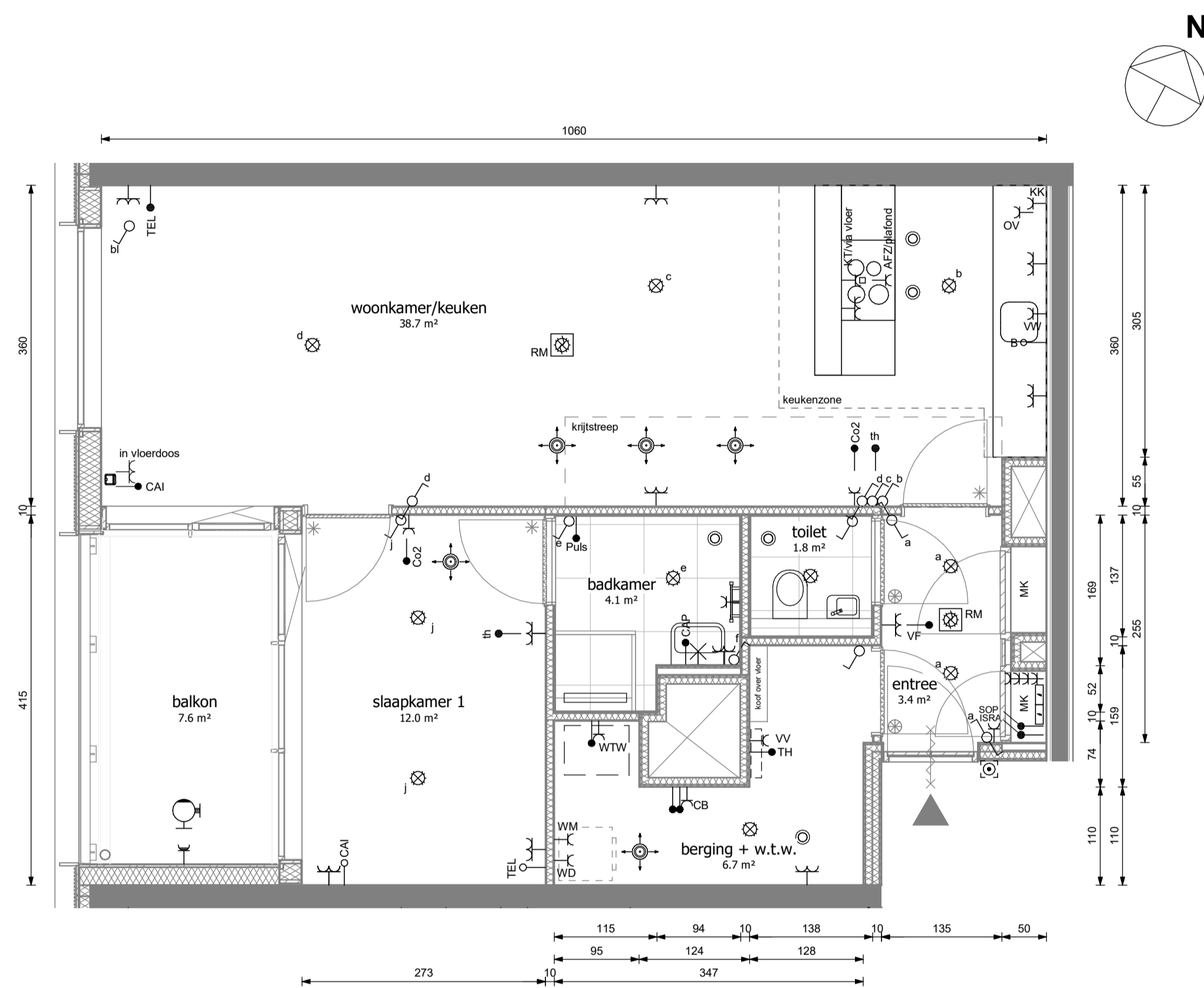
Type D2c schaal 1:50
