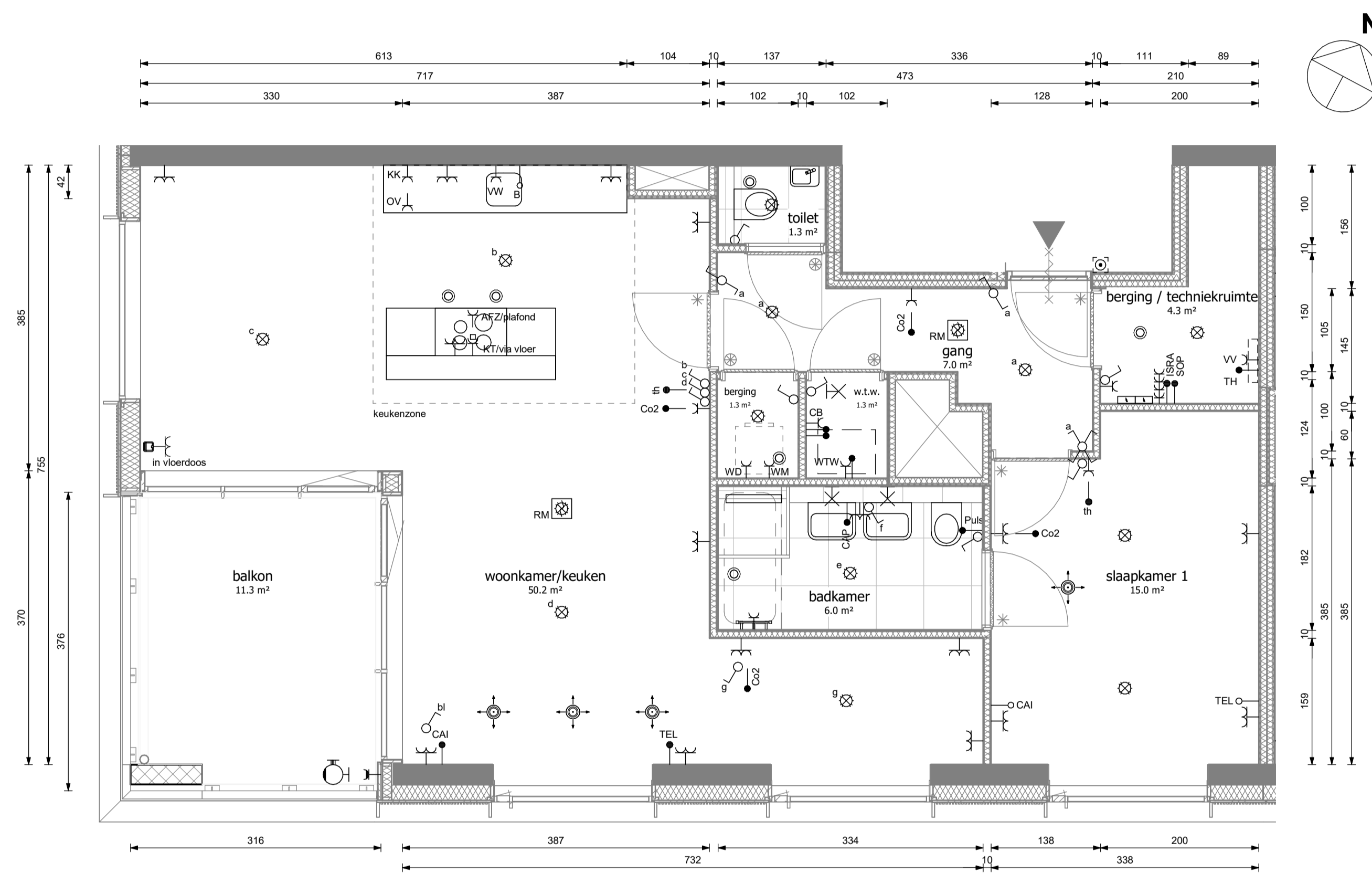
Type D1c schaal 1 : 50
